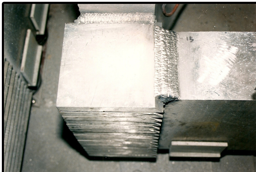
DC Rectifier Busbars 117VDC, 56kA 2x 90° Bend
